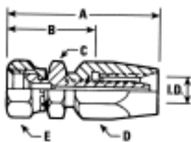
45° SAE SWIVEL
