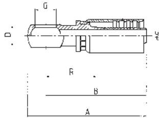
CODE BM METRIC BANJO DIN 7642
