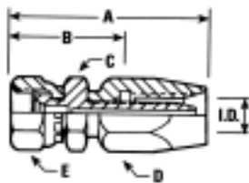
JIC 37° SWIVEL
